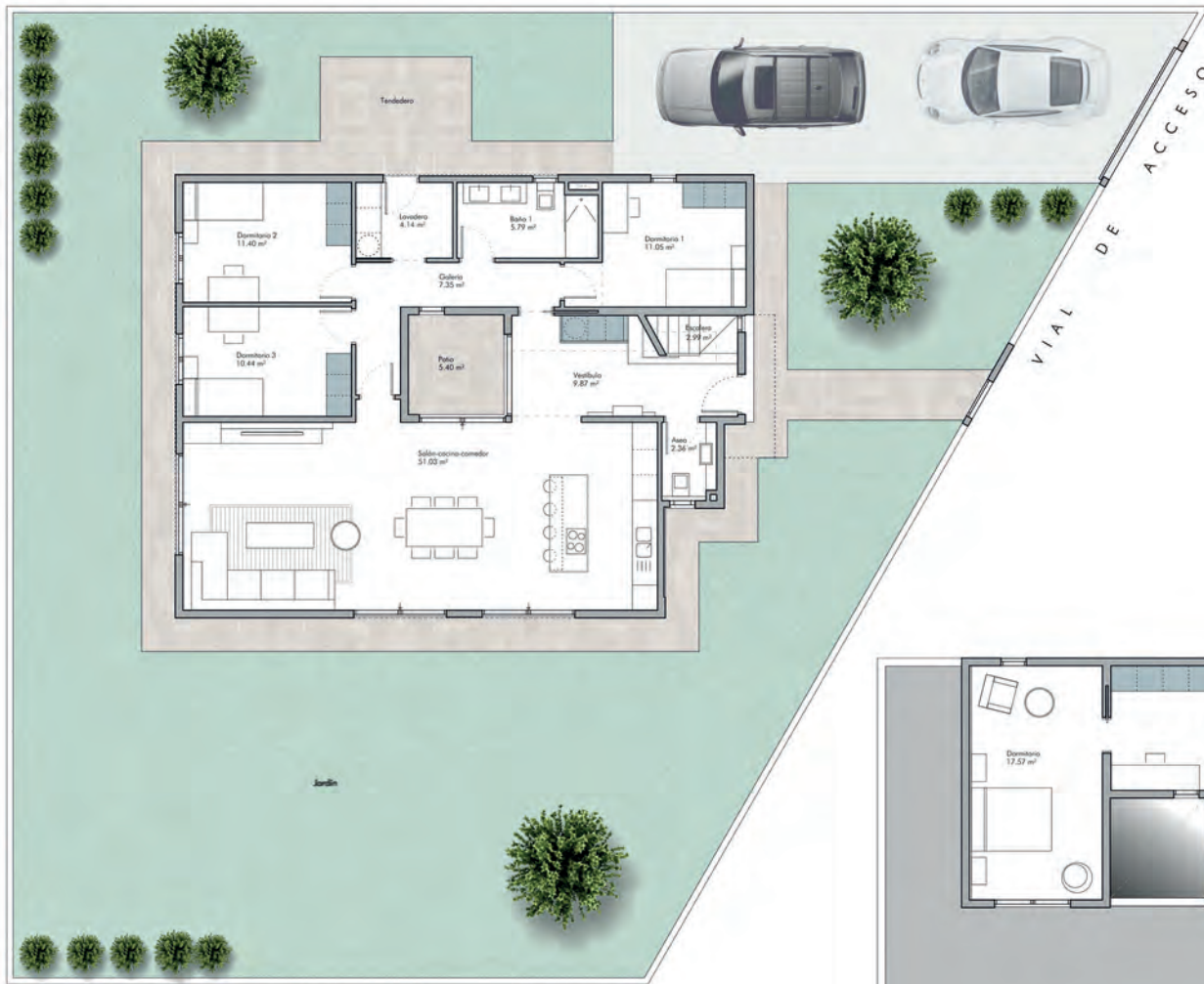
PLANTA BAJA
