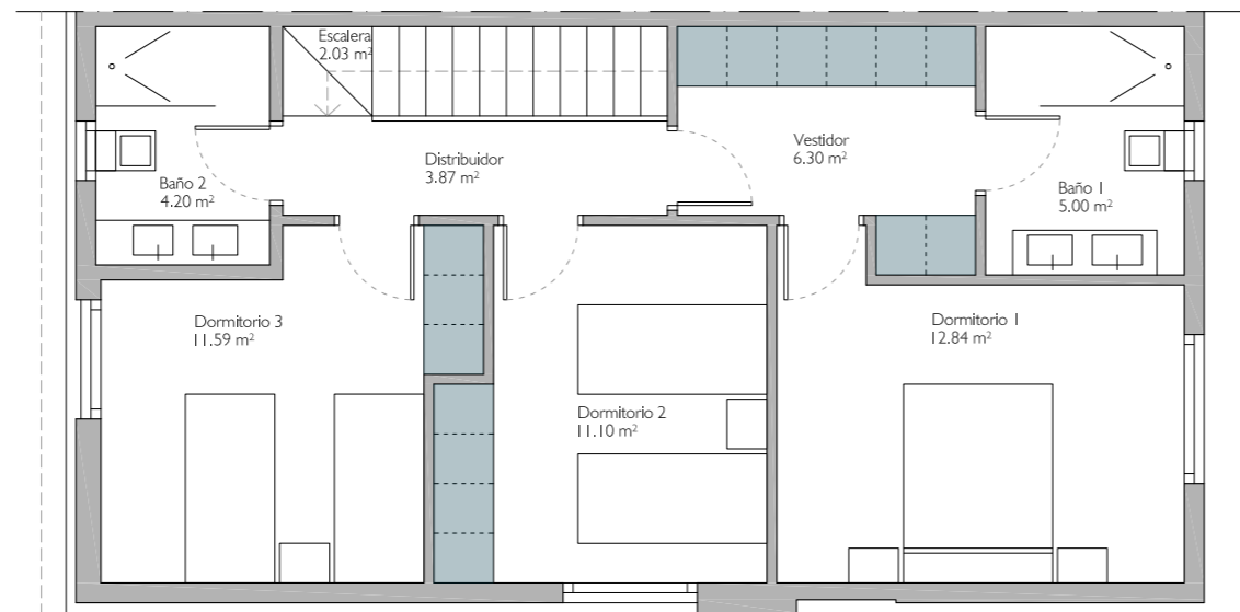
PLANTA ALTA
