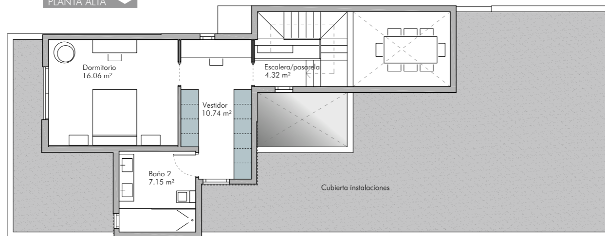
PLANTA ALTA
